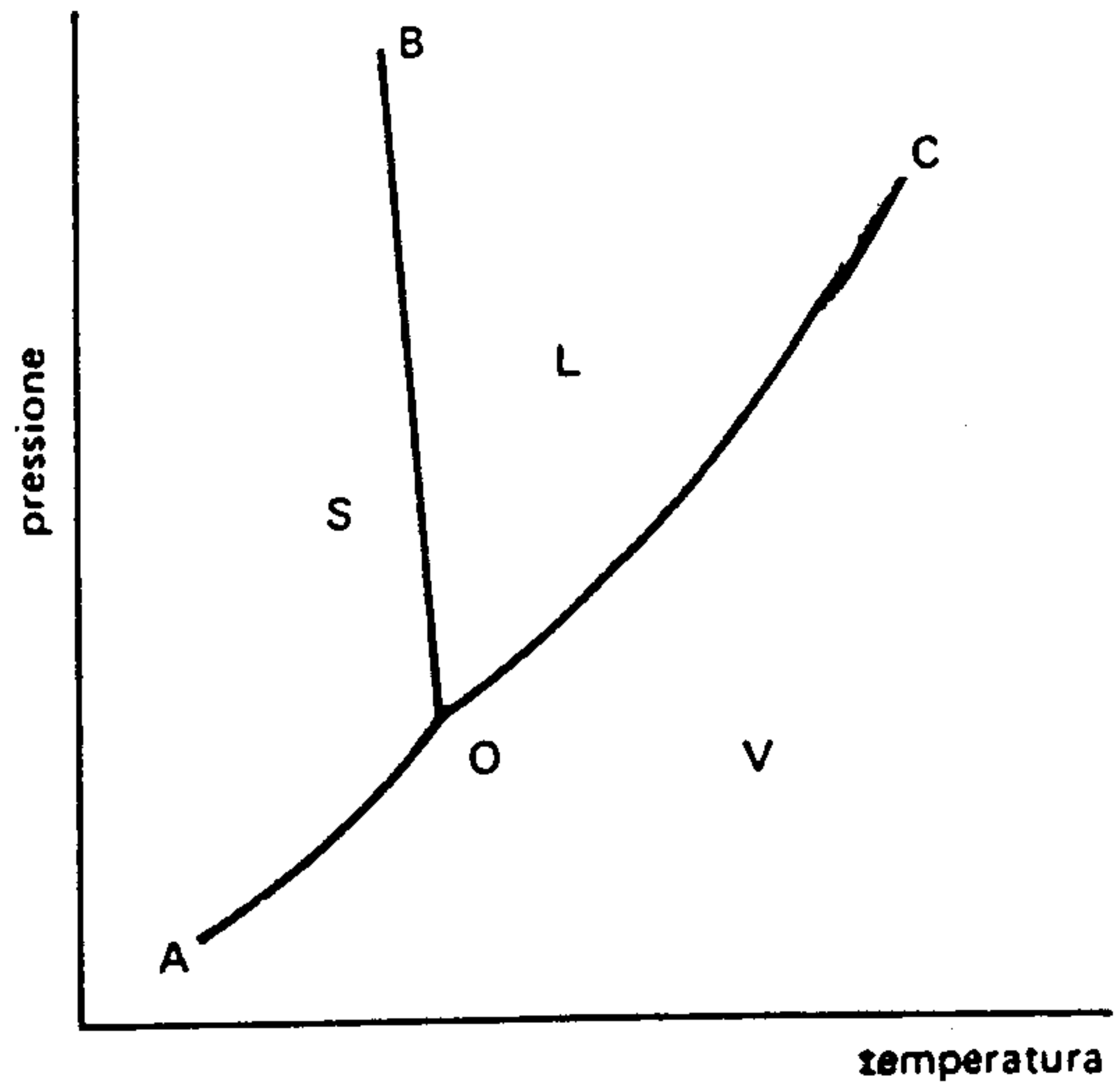
Figura 45 Diagramma di stato dell'acqua.
