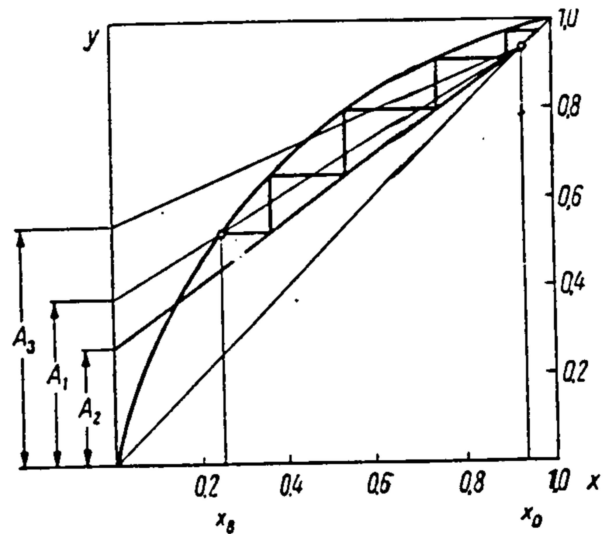
icolo grafico del numero di piatti teorici in caso di conten- tazione di distillato.
