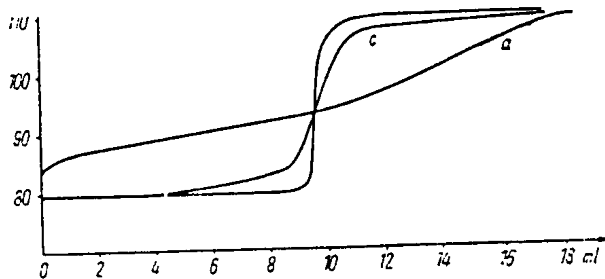
Fig. A.72. - Curve di ebollizione di una miscela benzolo-toluolo.
