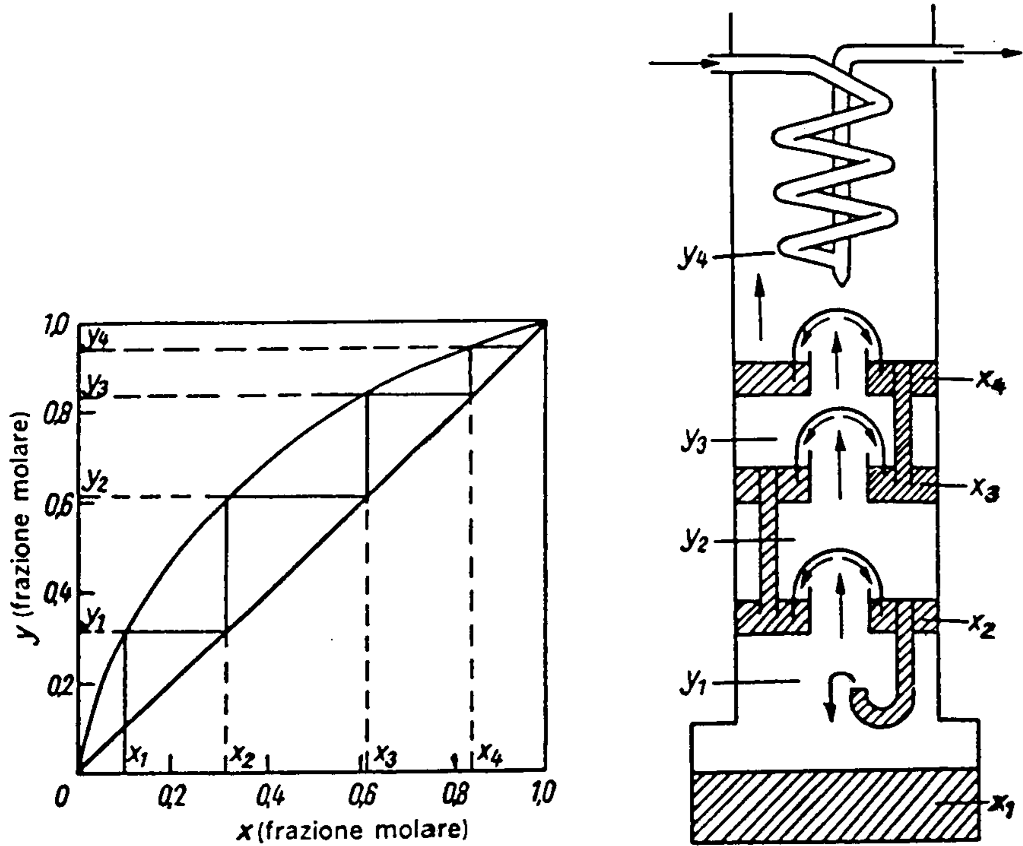
Fig. A.65. - Determinazione grafica del numero dei piatti teorici.
