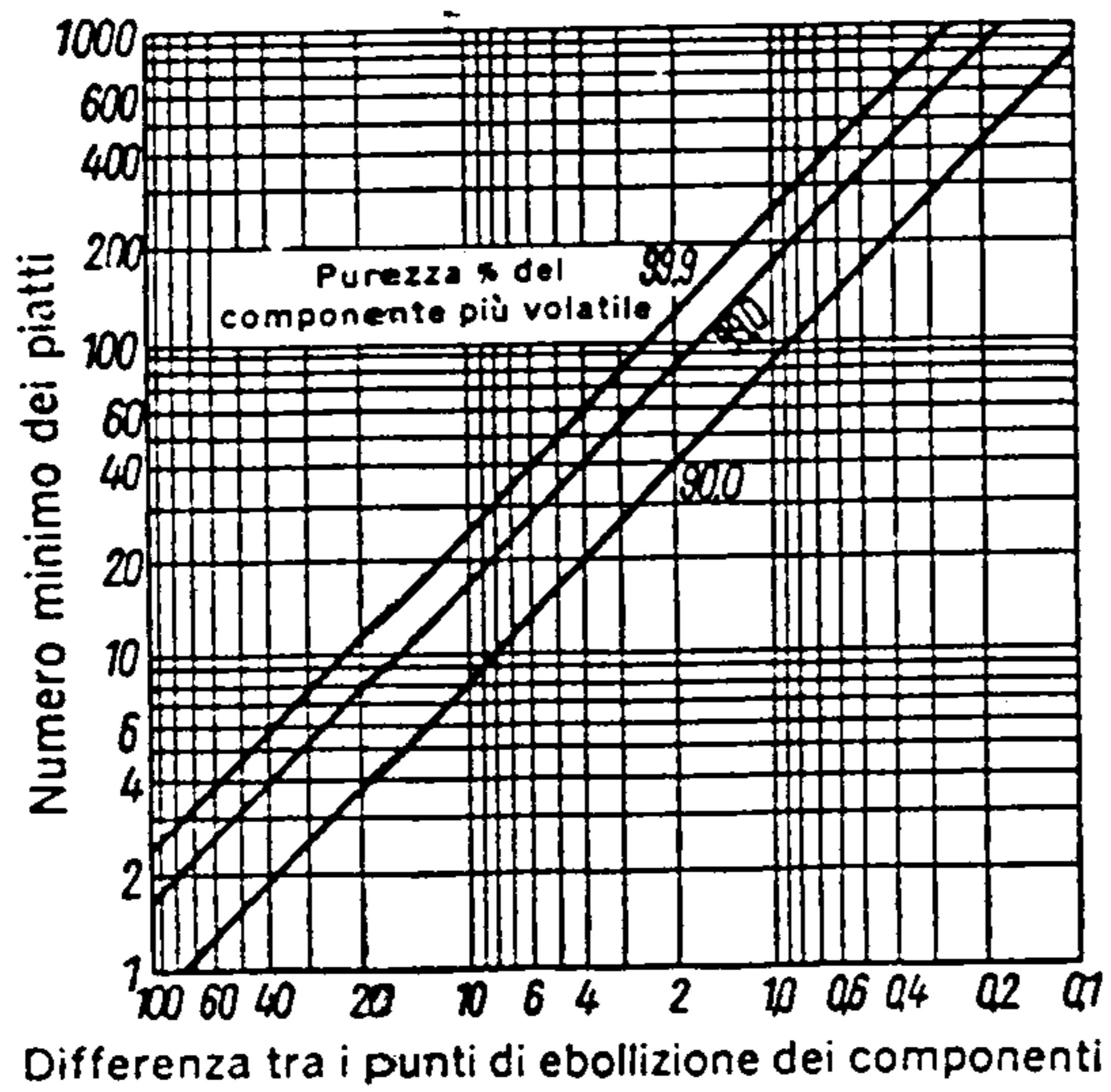
3. A.66. - Determinazione del numero dei piatti teorici in base alla differenza di punto di ebollizione dei componenti.
