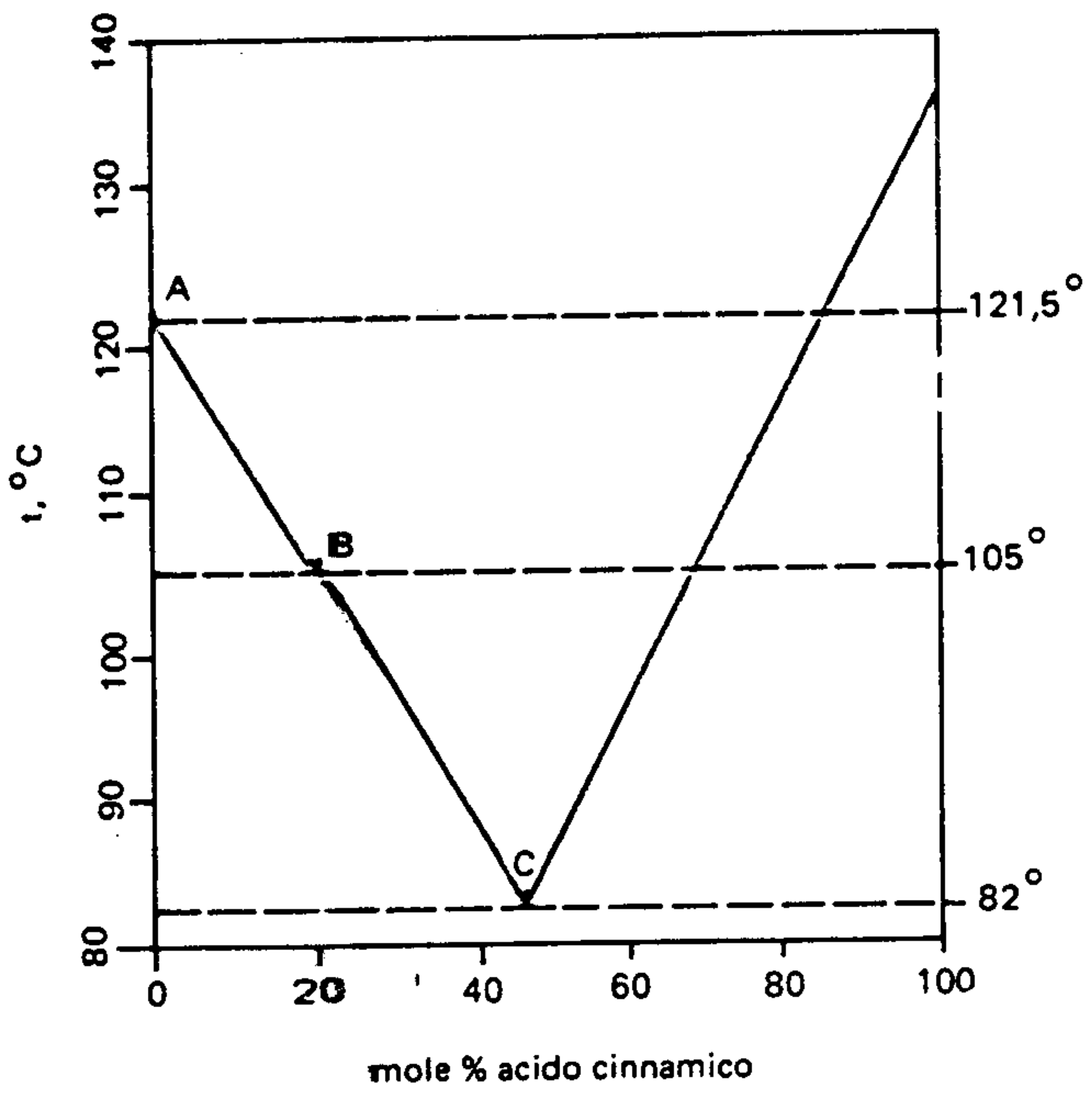
Figura 4.15 Sistema ac. benzoino-ac. cinnamico.
