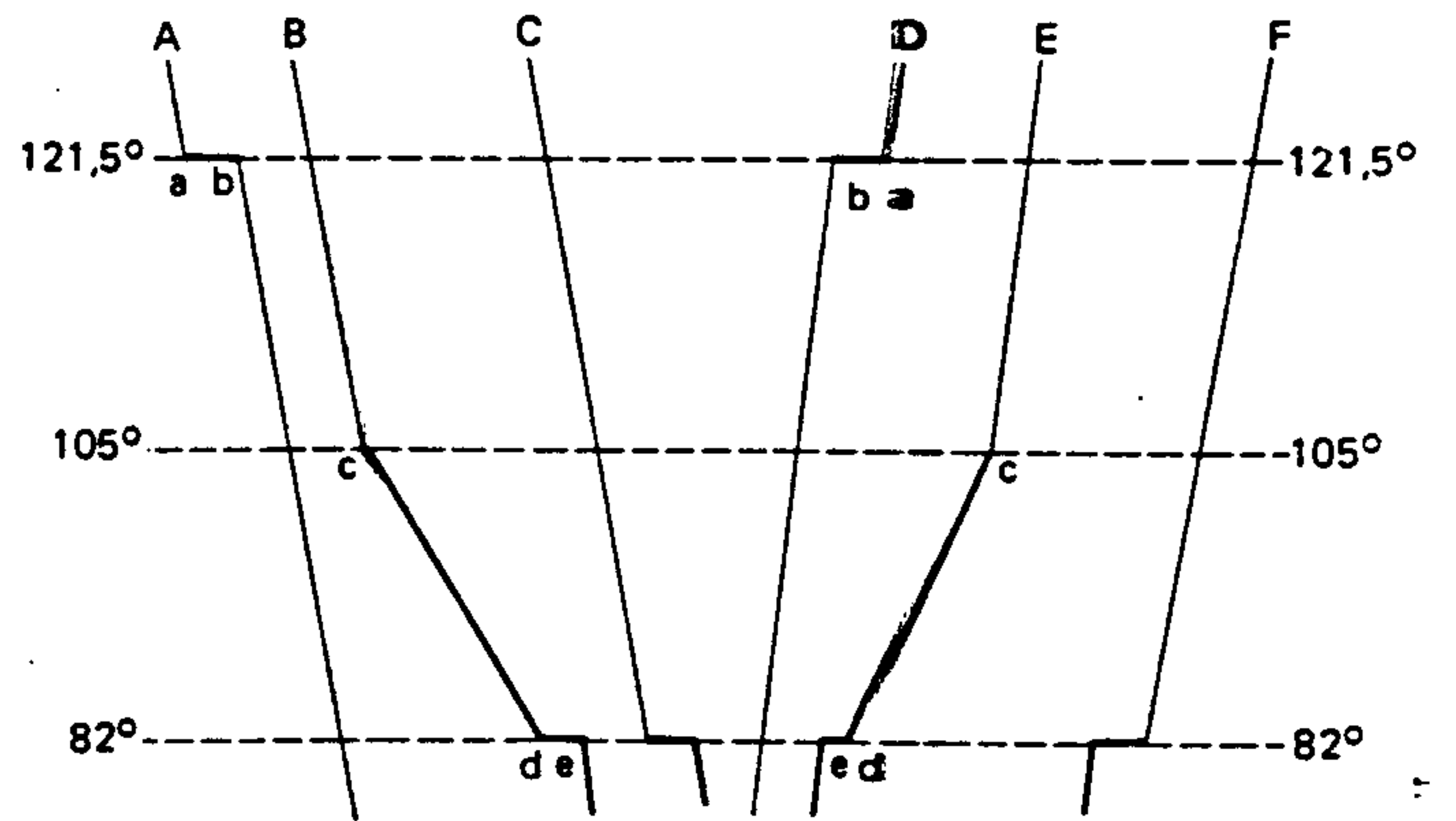
Figura 4.16 Curve di raffreddamento e riscaldamento relative al sistema di figura 4.15.
